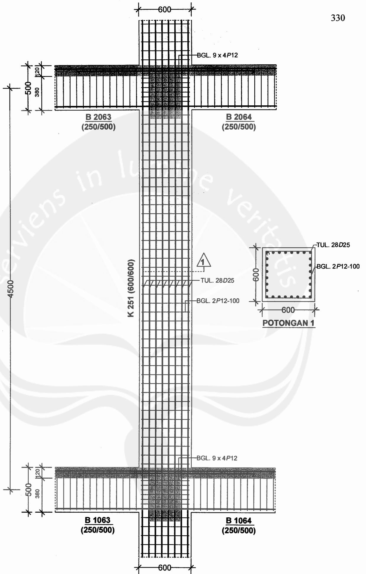
GAMBAR PENULANGAN KOLOM SKALA 1 : 25
