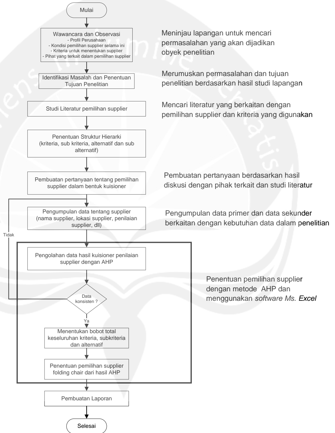
Gambar 3.1. Metodologi Penelitian
