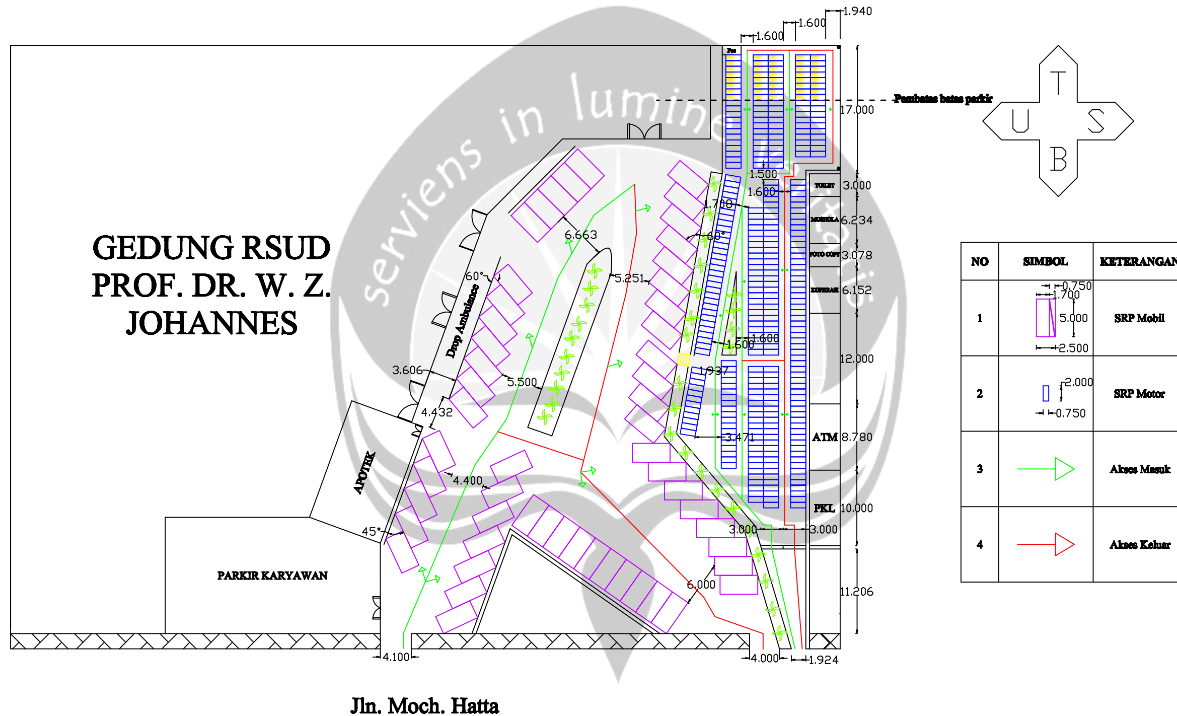
Lampiran 2.2. Gambar Penataan Parkir dengan Perubahan Sudut Parkir dan Memanfaatkan Lahan Sisi Selatan Rumah Sakit
