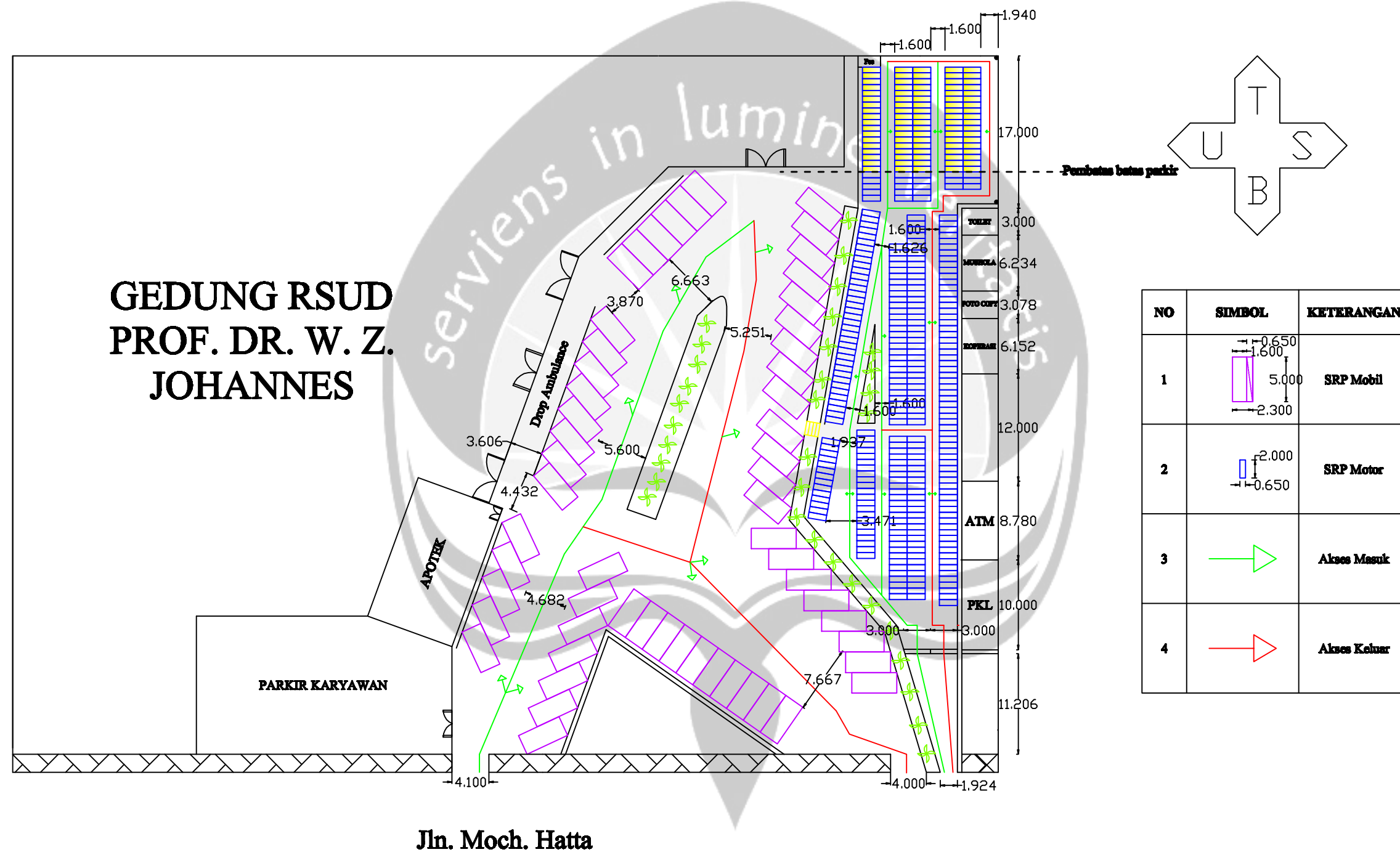
Lampiran 2.3. Gambar Penataan Parkir dengan Pengecilan SRP dan Memanfaatkan Lahan Sisi Selatan Rumah Sakit
