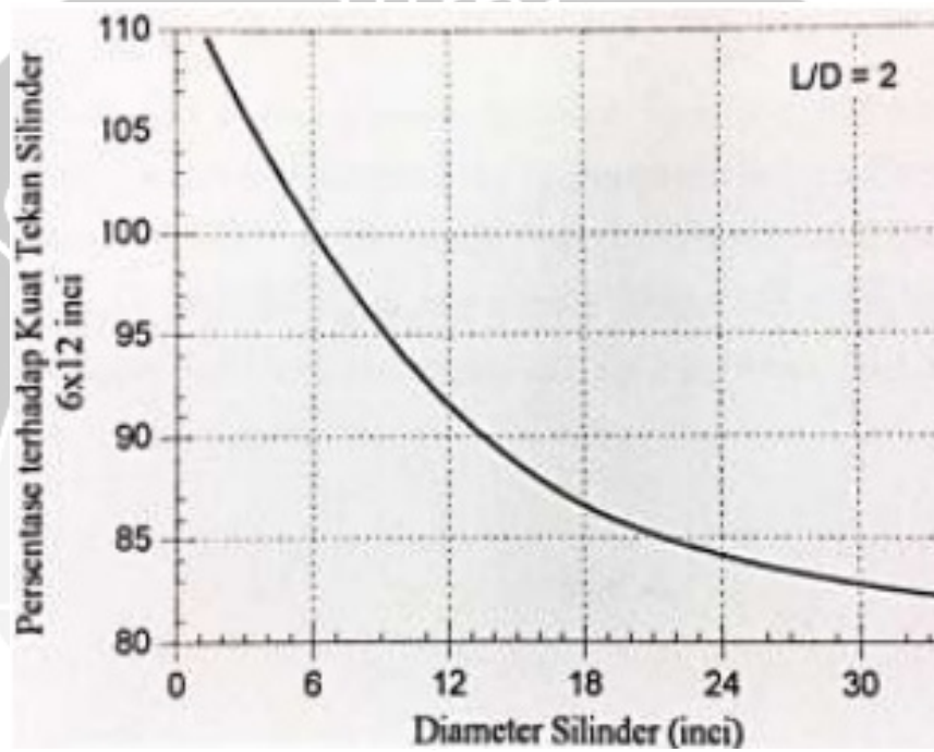
Gambar 3.1 Pengaruh Diameter Silinder Terhadap Kuat Tekan Beton
