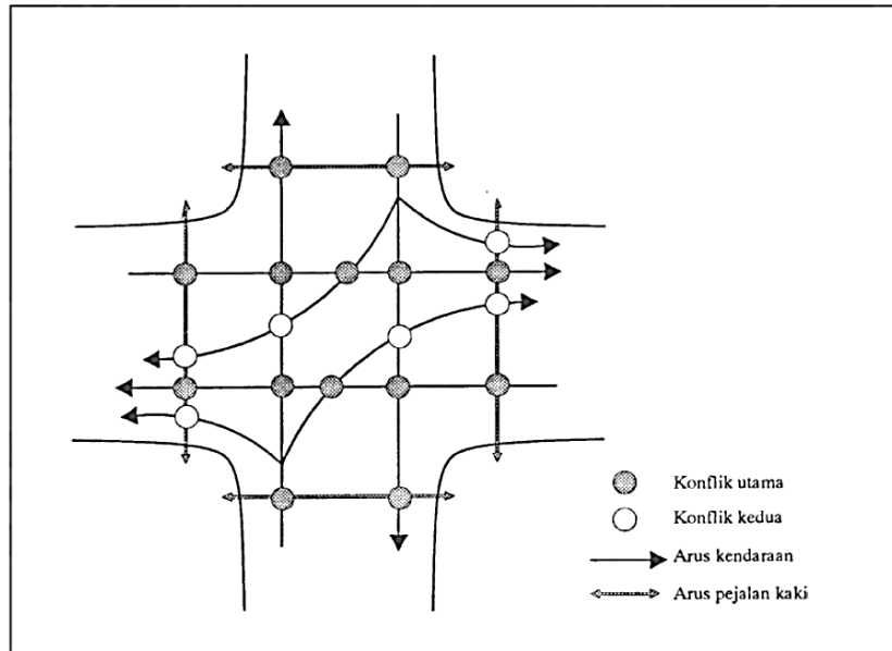
Gambar 2.3 Konflik Utama dan Kedua pada Simpang Bersinyal dengan Empat Lengan (MKJI, 1997)
