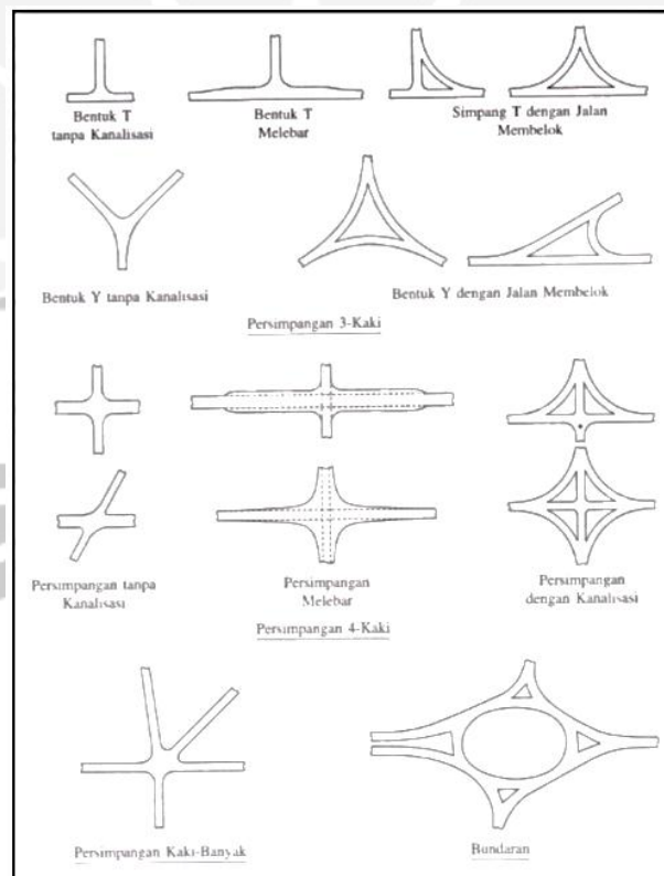
Gambar 2.1 Persimpangan Sebidang (Khisty dan Kent, 2005)
