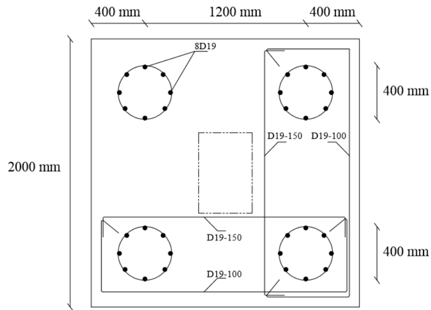
Detail Penulangan Pile Cap
