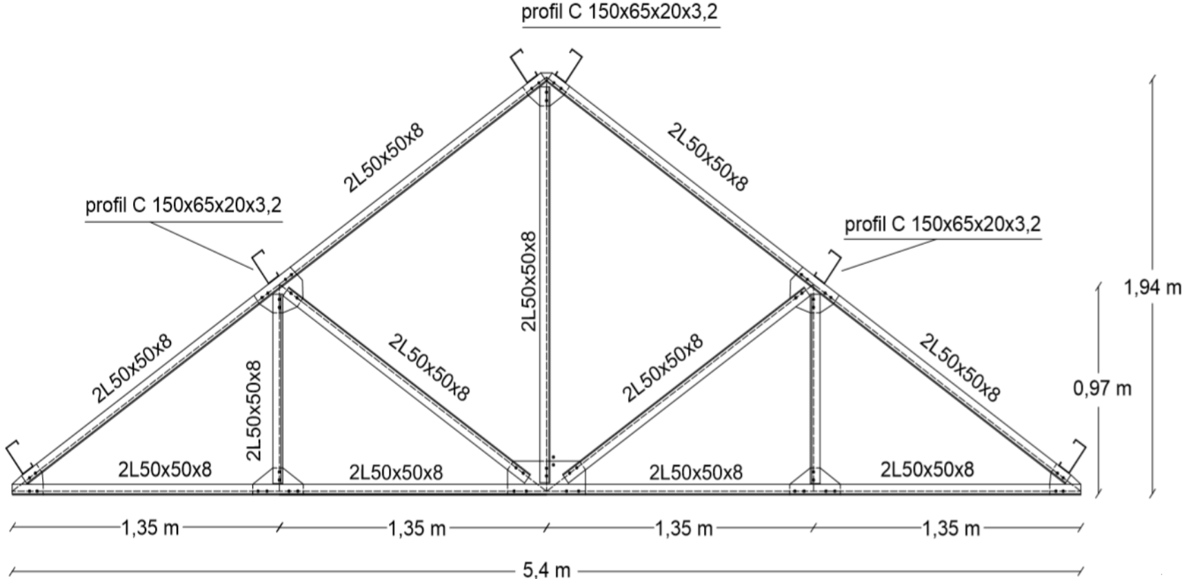
Gambar Kuda-Kuda
