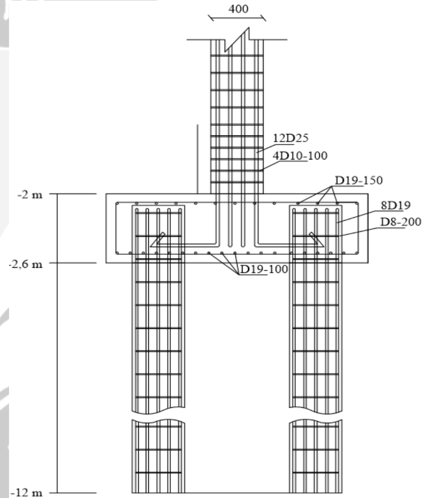
Detail Penulangan Tiang pancang
