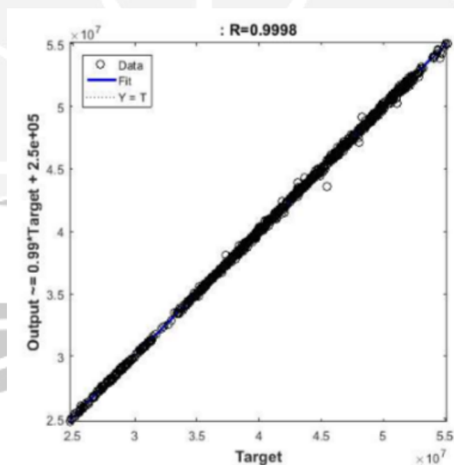
Gambar 4 Tingkat akurasi
