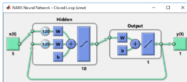
Gambar 3 Algoritma multi layer dengan perulangan
