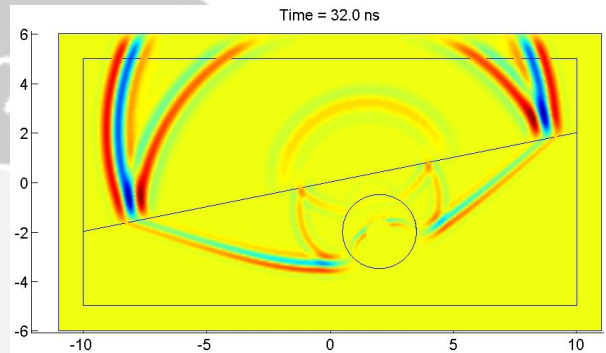
Gbr. 20 Perambatan gelombang elektromagnetik dalam media heterogen saat t=32 ns.
