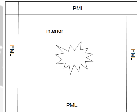
Gbr. 2 Syarat Batas PML.
