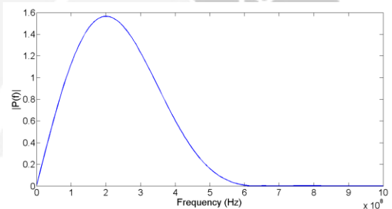
Gbr. 14 Spektrum source Blackman-Harris.
