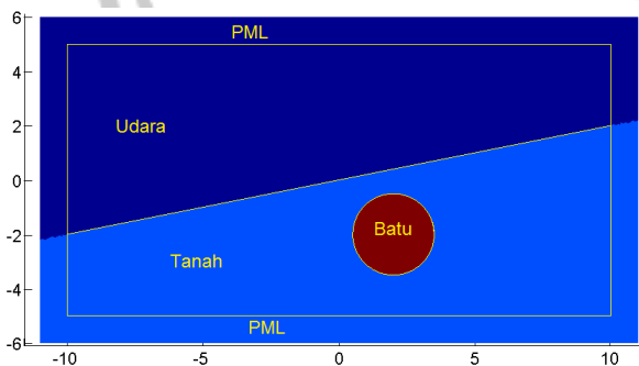
Gbr. 11 Domain ruang berikut distribusi material dan PML.
