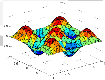
Gbr. 9 Amplitudo gelombang saat t = 0,8
