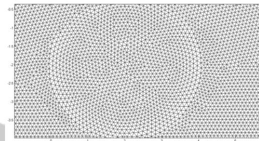
Gbr. 12 Mesh untuk area disekitar material batu.
