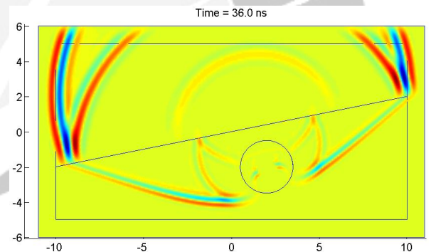
Gbr. 21 Perambatan gelombang elektromagnetik dalam media heterogen saat t=36 ns.
