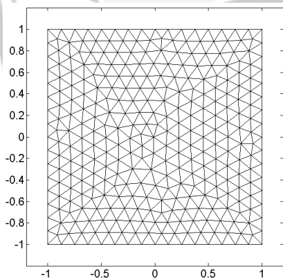
Gbr. 5 Mesh kotak 2-dimensi terdiri atas 568 elemen.
