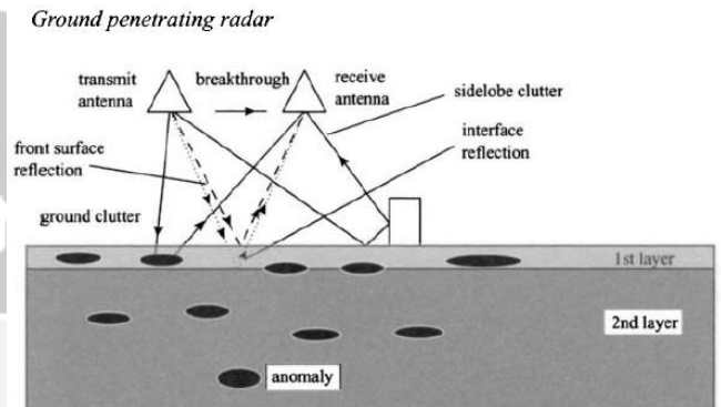
Gbr. 1 Prinsip kerja GPR [1].
