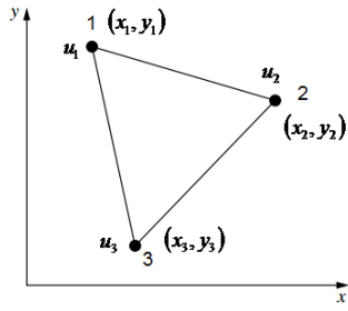
Gbr. 3 Elemen segitiga.
