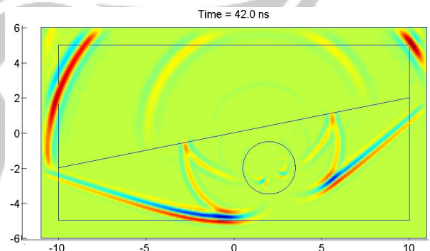
Gbr. 22 Perambatan gelombang elektromagnetik dalam media heterogen saat t=42 ns.
