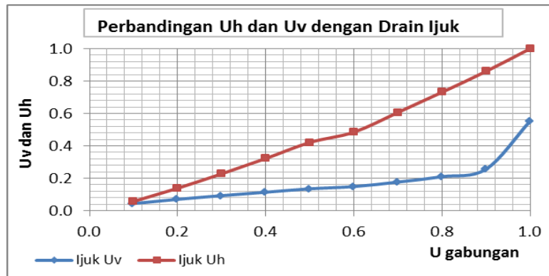
Gambar 4.9. Grafik Proses Konsolidasi arah vertikal dan horizontal drain ijuik
