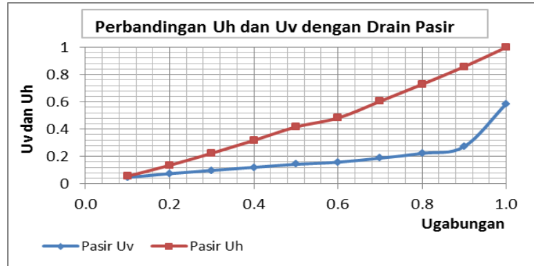
Gambar 4.8. Grafik Proses Konsolidasi arah vertikal dan horizontal drain pasir
