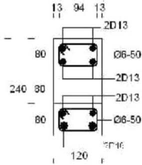
Gambar 6. Detil penulangan balok BOD1
