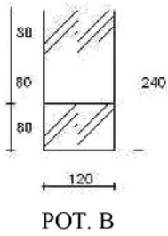
Gambar 4. Balok BOD3
