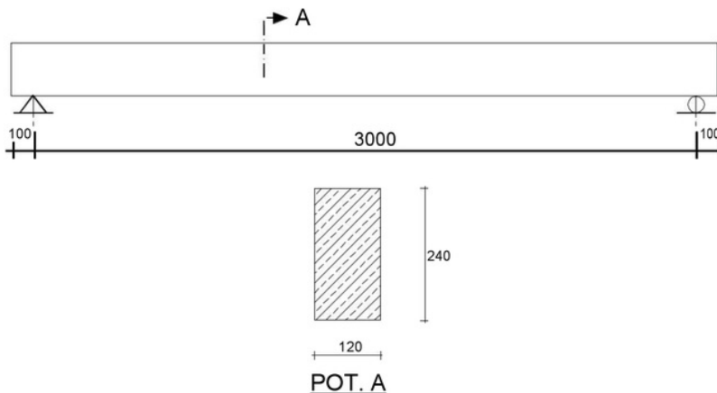
Gambar 1. Balok BSD
