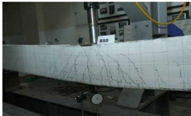
Gambar 10. Pola retak balok BSD
