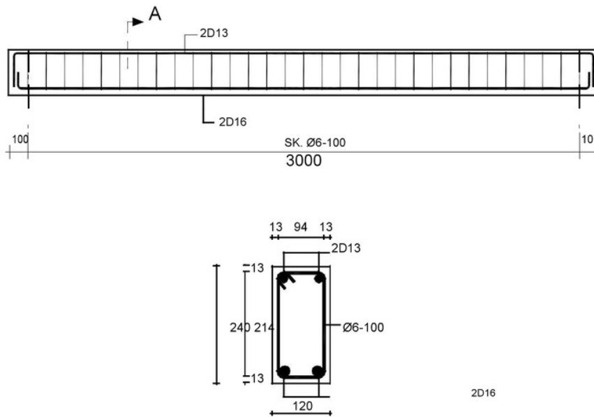
Gambar 5. Detil penulangan balok BSD
