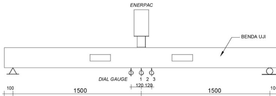
Gambar 9. Setup pengujian balok
