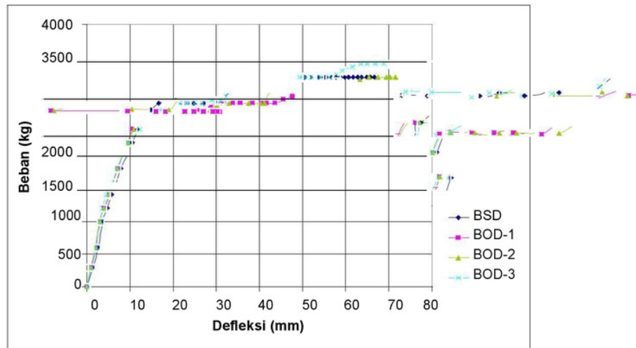
Gambar 17. Kurva beban-defleksi balok uji
