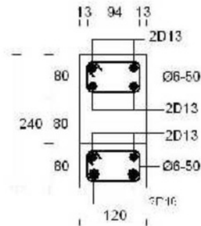
Gambar 7. Detil penulangan balok BOD2
