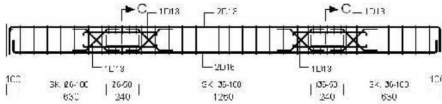
Gambar 6. Detil penulangan balok BOD1
