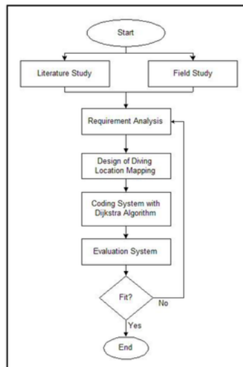
Fig. 1. Metodoly
