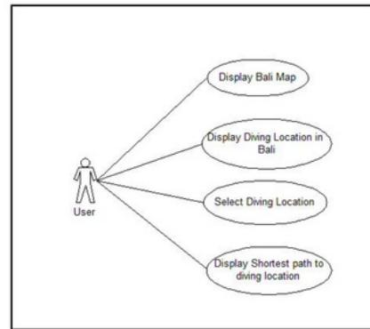
Fig. 3. Usecase Diagram
