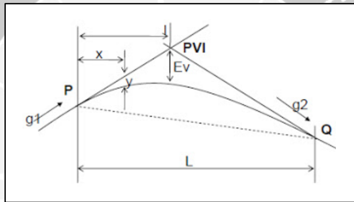
Gambar 3.13 Tipikal lengkung vertikal bentuk parabola Sumber : Hendarsin (2000)
