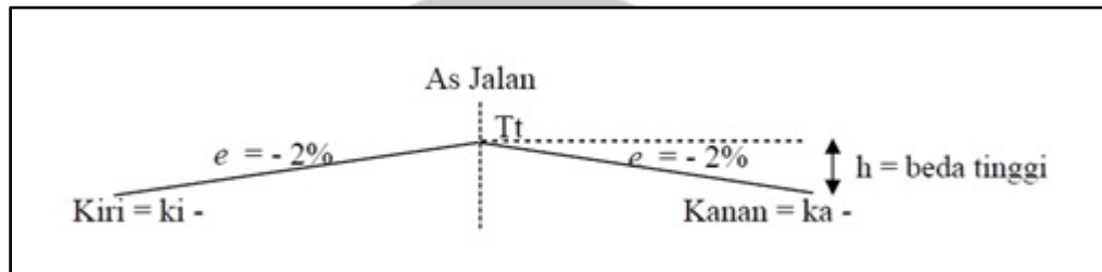
Kemiringan normal pada bagian jalan lurus
