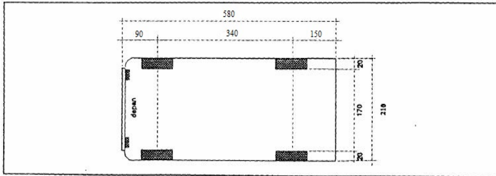
Gambar 3.1 Dimensi Kendaraan Kecil
