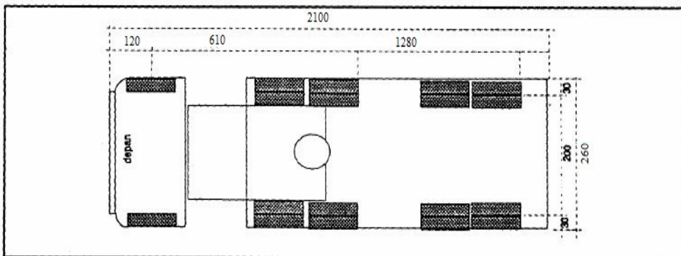
Gambar 3.3 Dimensi Kendaraan Besar
