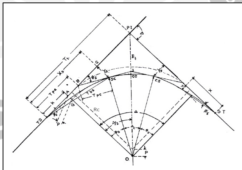
Gambar 3.7 Lengkungan Spiral - Circle - Spiral
