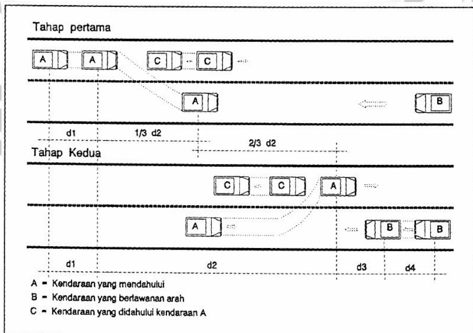
Gambar 3.4 Jarak pandang mendahului
