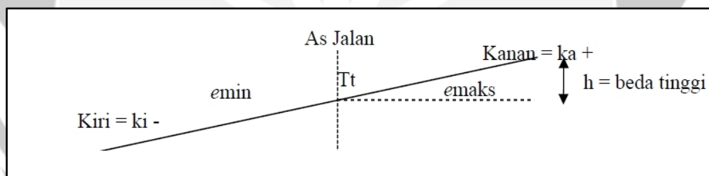
Kemiringan melintang pada tikungan pada tikungan belok
