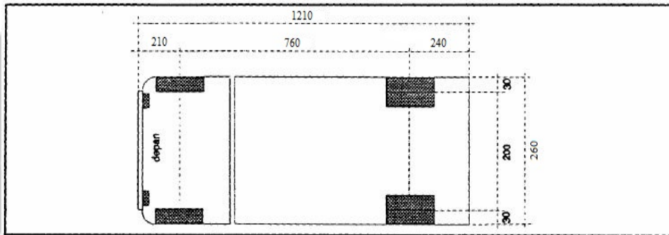
Gambar 3.2 Dimensi Kendaraan Sedang
