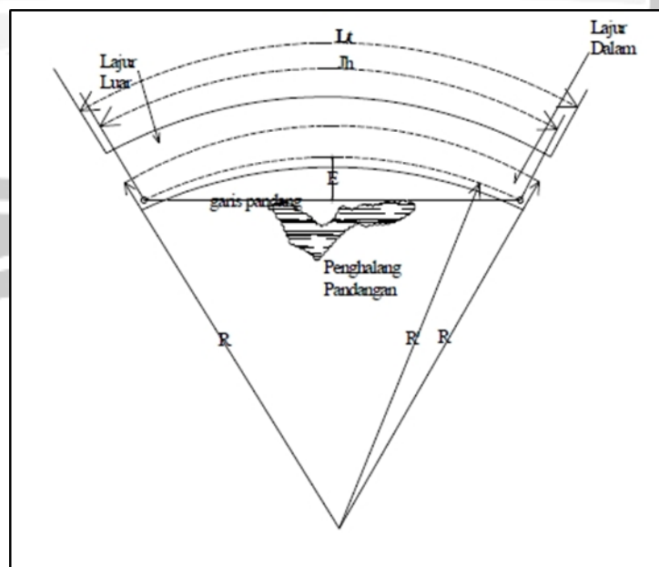
Gambar 3. 5 Daerah bebas samping di tikungan, untuk Jh < Lt . Sumber : Tata Cara Perencanaan Geometrik Jalan Antar Kota No.038/TBM/1997.
