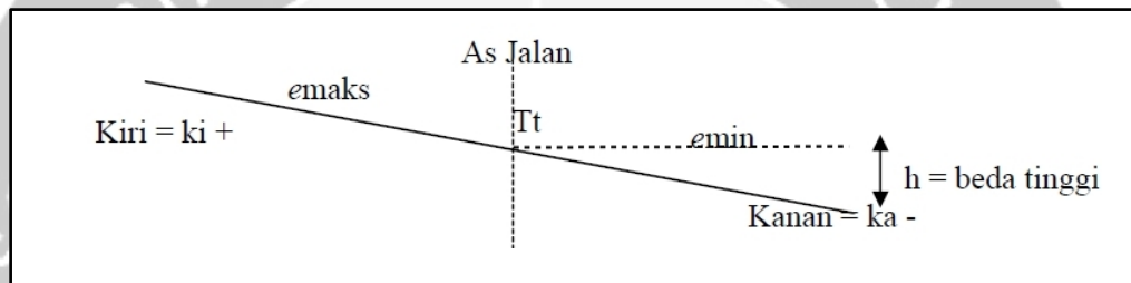
Kemiringan jalan pada tikungan belok kanan
