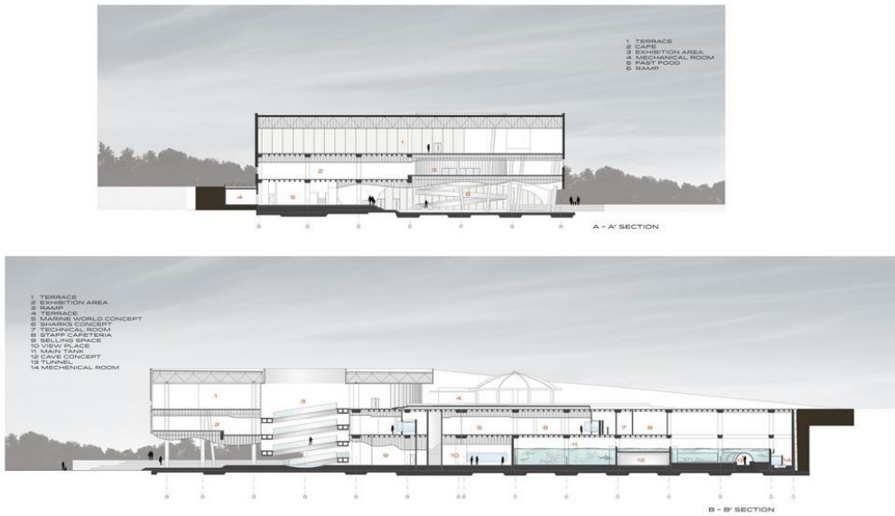
Gambar 2.25 Potongan Antalya Aquarium Sumber : www.archdaily.com
