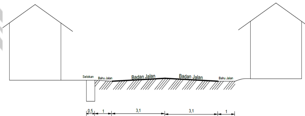
Gambar 6.1 Potongan Melintang Pelebaran Jalan Andi Mappanyukki
