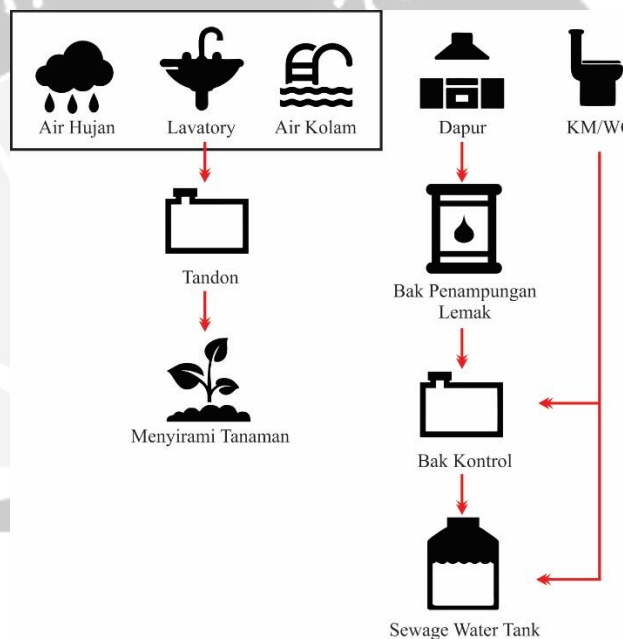
Skema 6.2: Skema Sistem Distribusi Air Kotor (Sumber: Analisis Pribadi, 2017)
