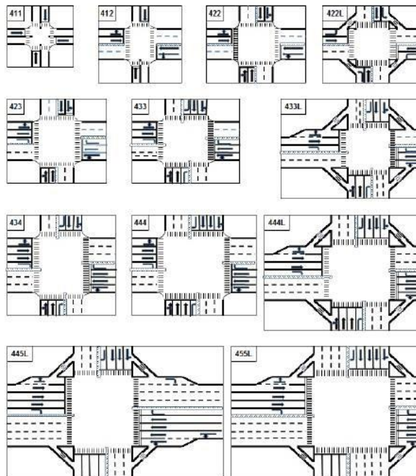
Gambar 3.1 Tipikal Geometrik Simpang Empat
