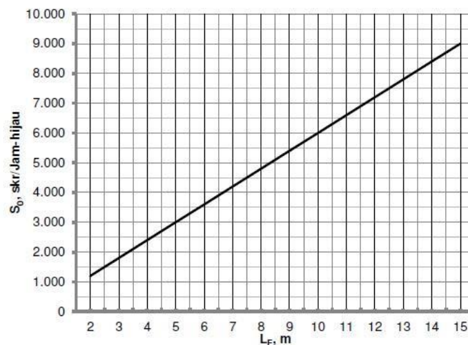
Gambar 3.3 Arus Jenuh Dasar Pendekat Terlindung (Tipe P)
