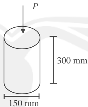
Gambar 3.1 Uji Kuat Tekan Beton pada Benda Uji Silinder
