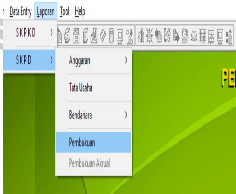
Gambar 2.95. Toolbar SIMDA
