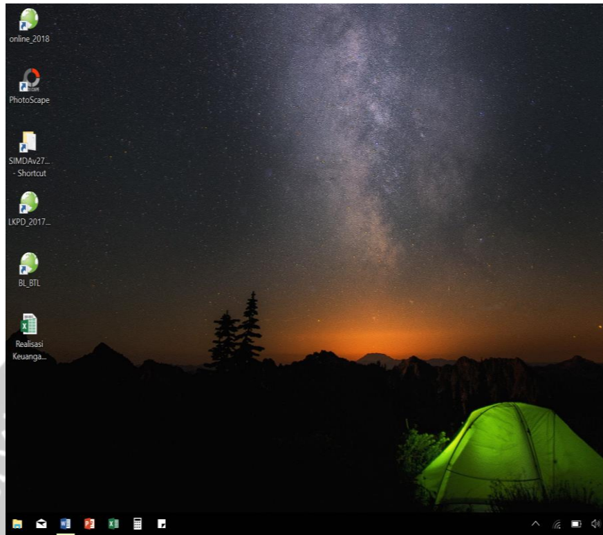
Gambar 2.3. Aplikasi SIMDA
