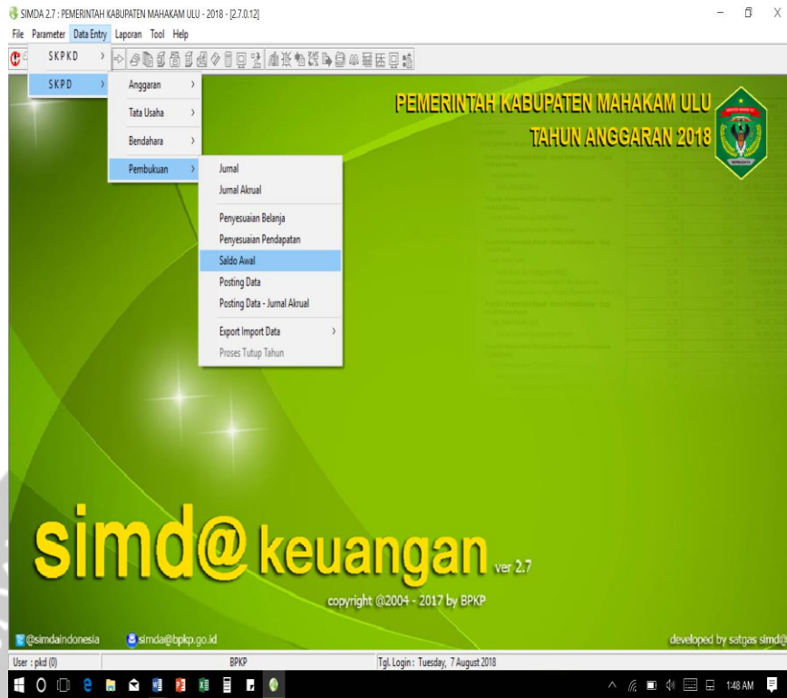
Gambar 2.5. Toolbar SIMDA
