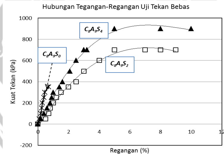
Gambar 4. Hasil Uji Tekan Bebas : Kuat tekan vs. regangan aksial
