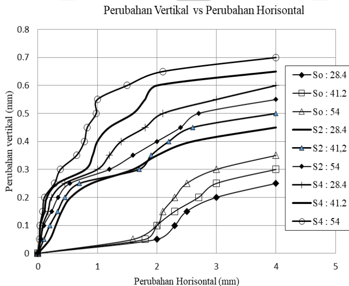
Gambar 2. Hubungan antara perubahan vertikal dengan perubahan lateral
