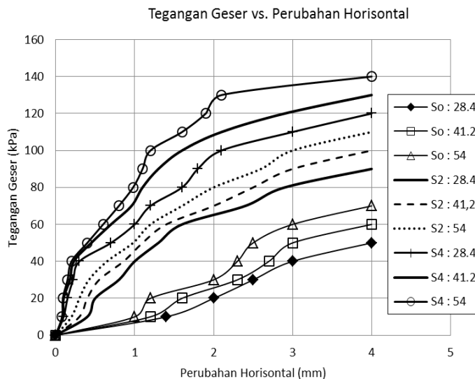
Gambar 1. Hubungan antara tegangan geser dengan perubahan lateral
