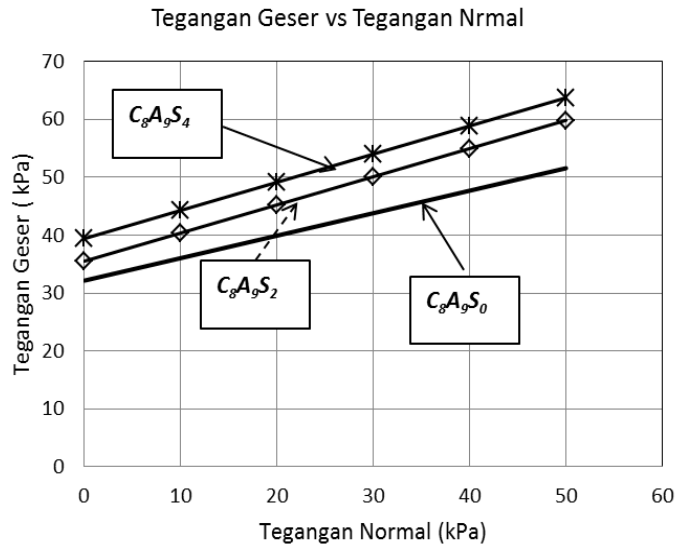
Gambar 3. Hasil uji geser langsung Tanah + semen + AAT + serat polyester
