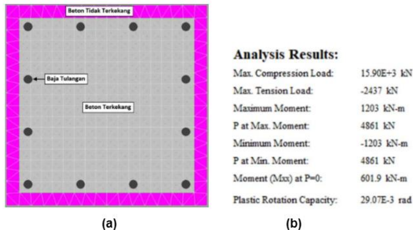
Gambar 4. Tampang kolom dan hasil analisis tampang: (a) Kolom 600x600mm dan (b) Hasil analisis XTRACT
