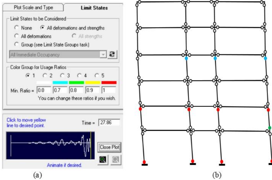
Gambar 15. Hasil analisis dinamik nonlinier struktur terhadap gempa Padang 2009 yang telah disesuaikan ke level gempa MCE: (a) Plot respon SRBPMK; (b) Hasil animasi sesaat sebelum analisis dihentikan (setelah 27,86 detik - arah H1)
