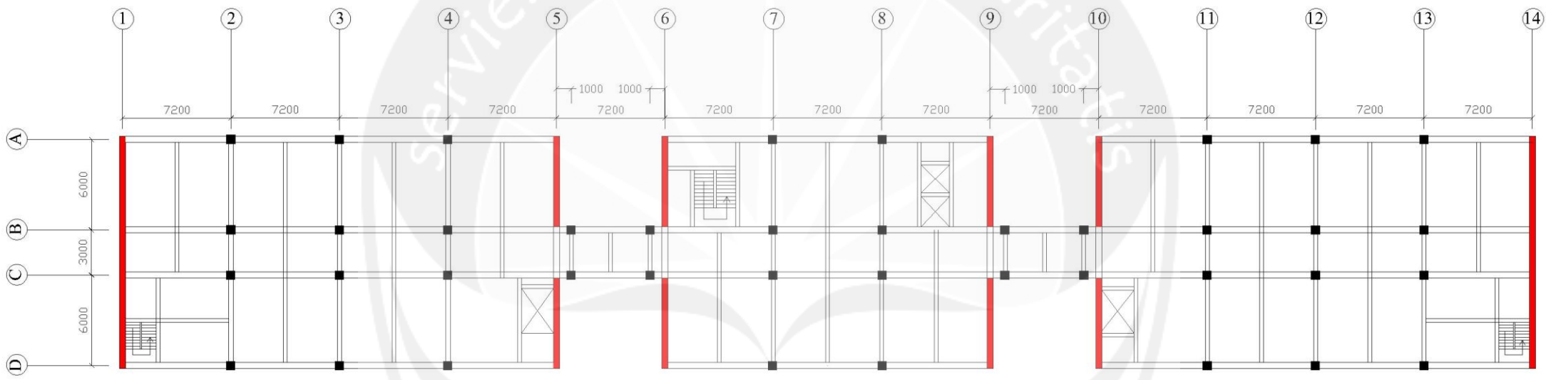
DENAH BALOK KOLOM LANTAI 1, 2, 3, & 4 SKALA 1:400
