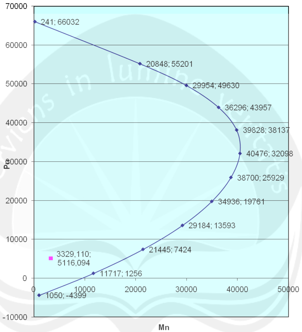
Digram Interaksi Dinding Geser
