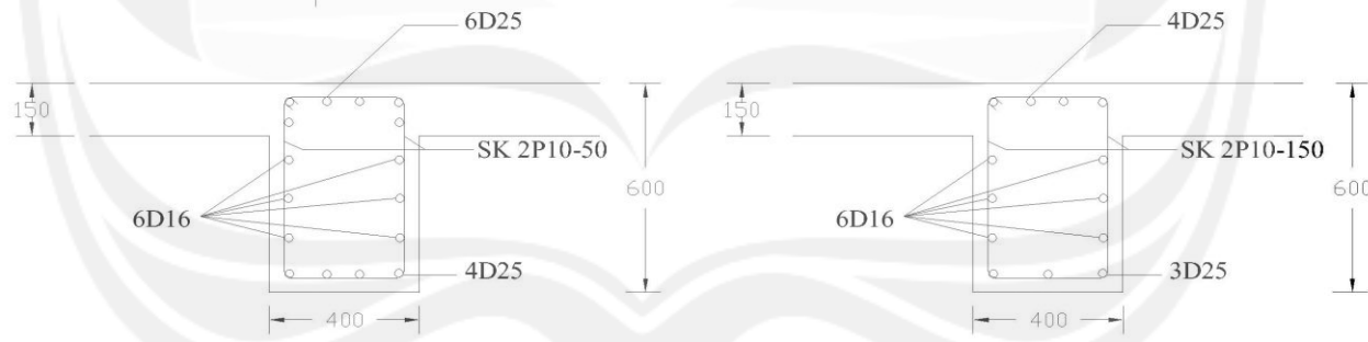
POTONGAN 1-1 SKALA 1 : 20
