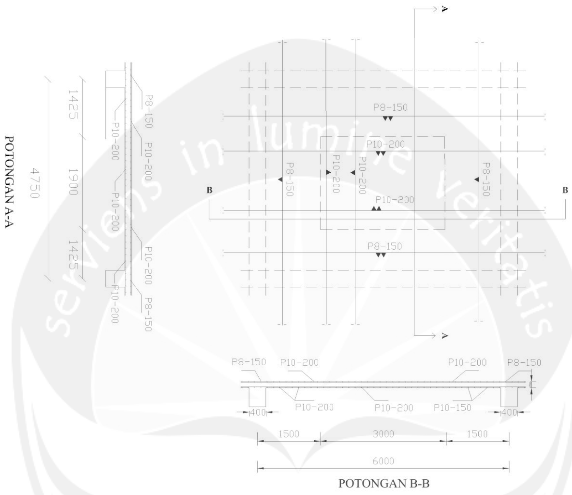
GAMBAR PENULANGAN PELAT DUA ARAH PADA ATAP SKALA 1 : 75
