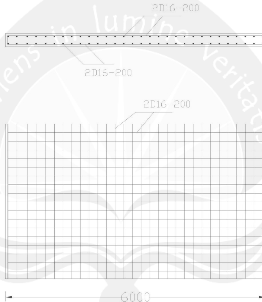
PENULANGAN DINDING GESER Skala 1 : 60
