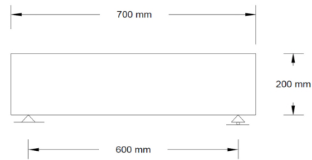
Gambar 2. Benda uji balok beton
