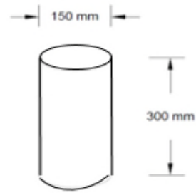
Gambar 1. Benda uji silinder
