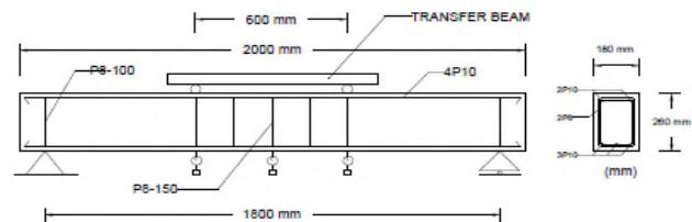
Gambar 3. Detil penulangan balok
