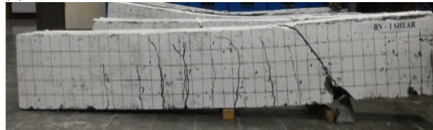
(b) Pola retak balok BS-2
