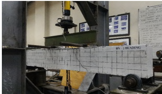
Gambar 4. Setup benda uji balok beton bertulang
