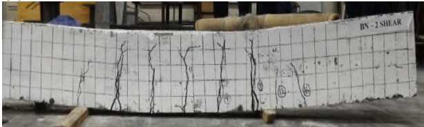
(b) Pola retak balok BS-1
