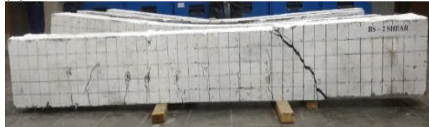
Gambar 7. Pola retak balok BN-1 dan BS-2.
