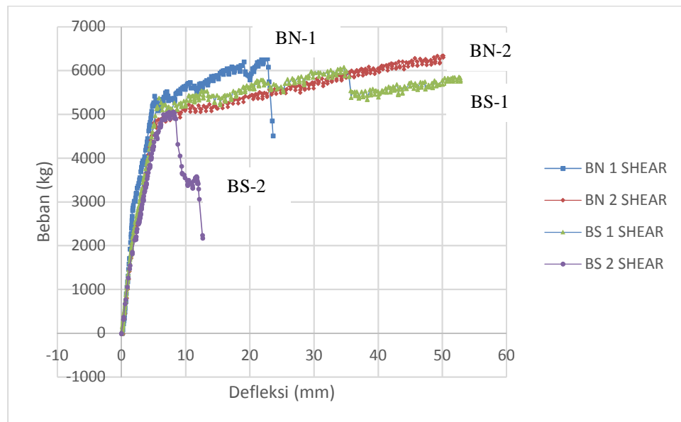
Gambar 6. Hubungan beban-defleksi balok beton bertulang memadat sendiri tanpa dan dengan serat polypropylene
