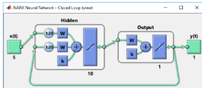
Gambar 3 Algoritma multi layer dengan perulangan
