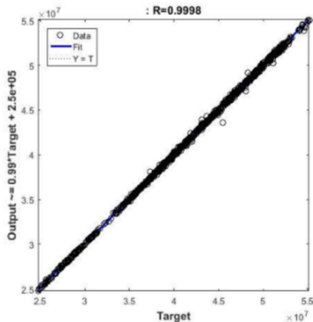
Gambar 4 Tingkat akurasi
