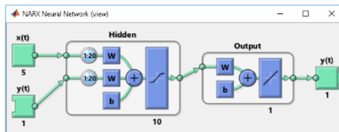
Gambar 2 Algoritma multi layer
