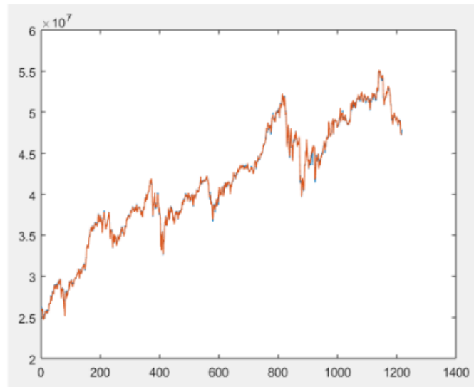
Gambar 5 Perbandingan hasil permalan dengan data asli
