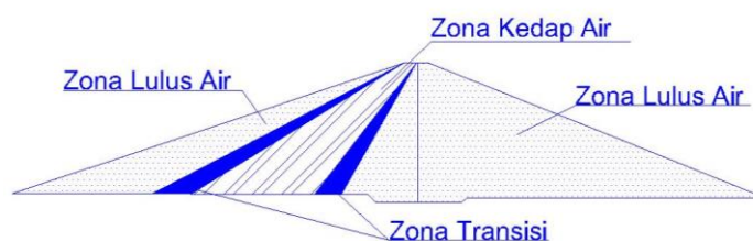
Gambar 3.2 Bendungan Urugan Zonal dengan Inti Kedap Air Miring
