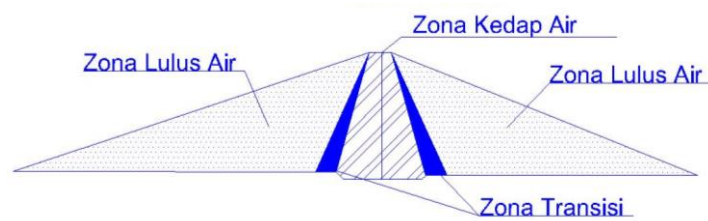
Gambar 3.3 Bendungan Urugan Zonal dengan Inti Kedap Air Tegak
