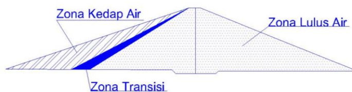
Gambar 3.1 Bendungan Urugan Zonal dengan Tirai Kedap Air
