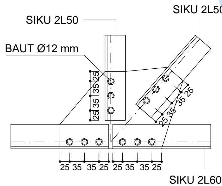
DETAIL B SAMBUNGAN BAUT 1:2,5
