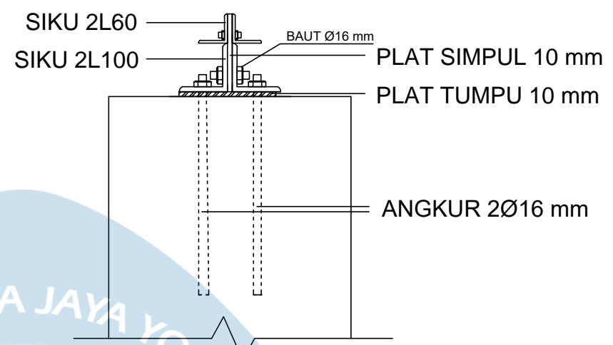
POTONGAN A 1:5
