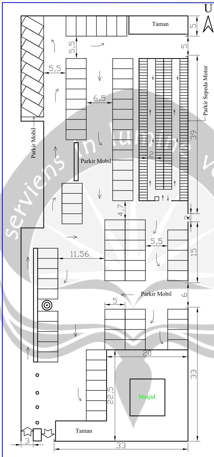
Gambar 5.15. Denah Parkir Rumah Sakit Islam Klaten
