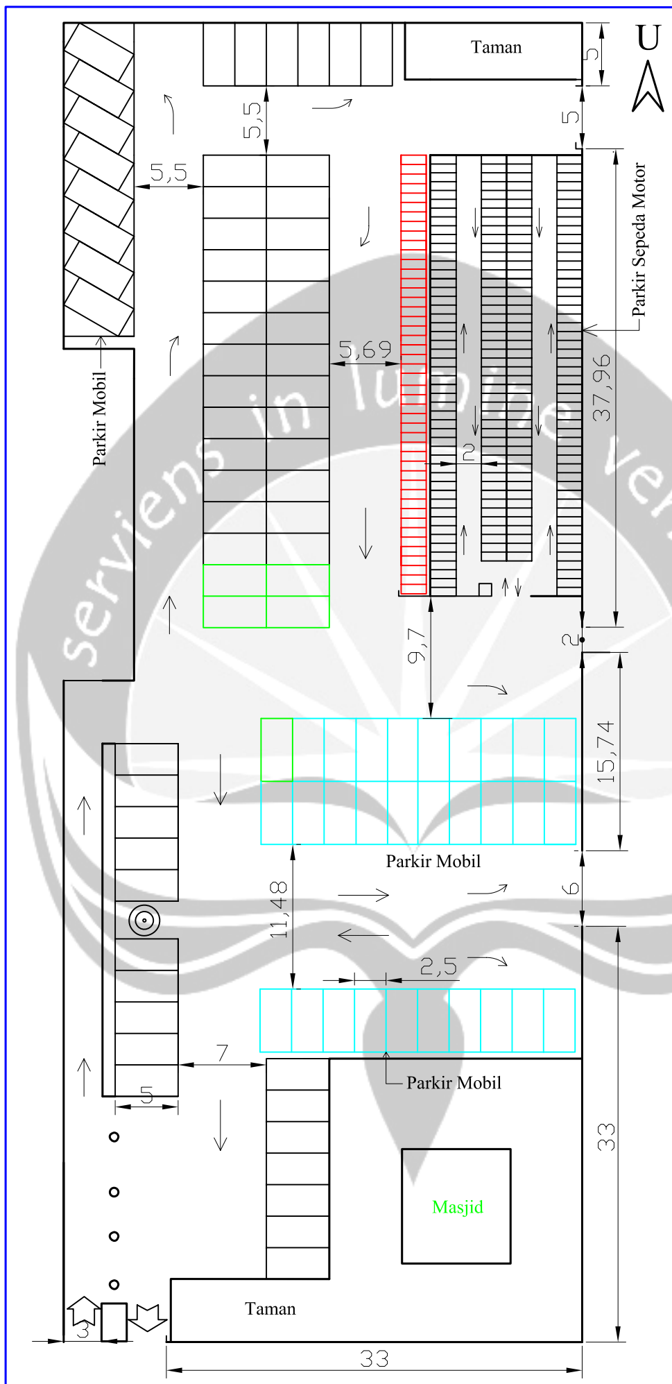
Gambar 5.16. Desain Alternatif Parkir Rumah Sakit Islam Klaten
