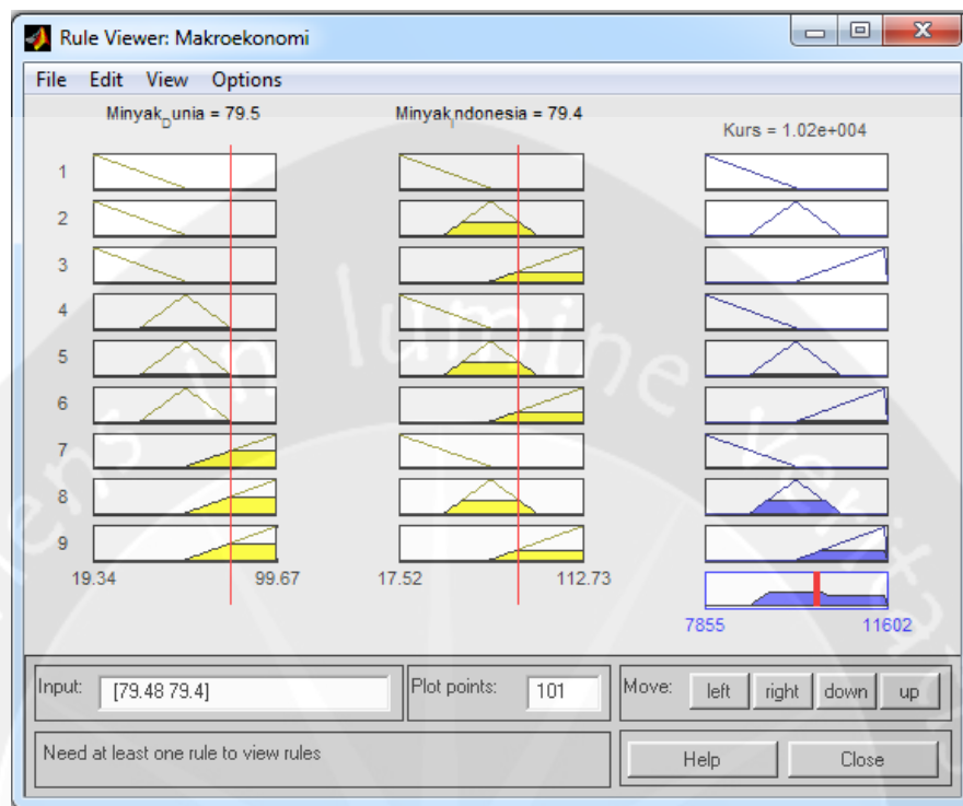
Lampiran 1.51 Deffuzifikasi tahun 2010
