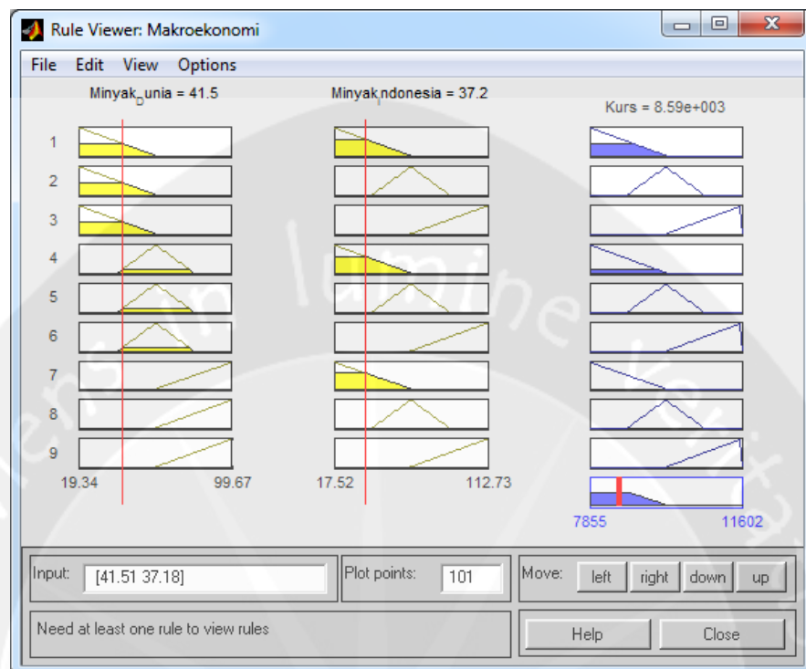
Lampiran 1.45 Deffuzifikasi tahun 2004
