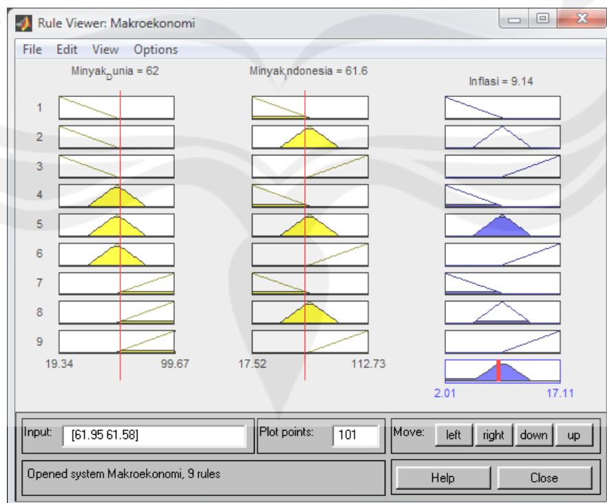
Lampiran 1.16 Deffuzifikasi tahun 2009
