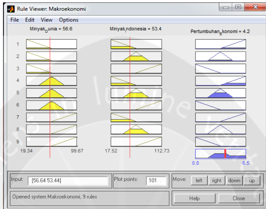
Lampiran 1.29 Deffuzifikasi tahun 2005
