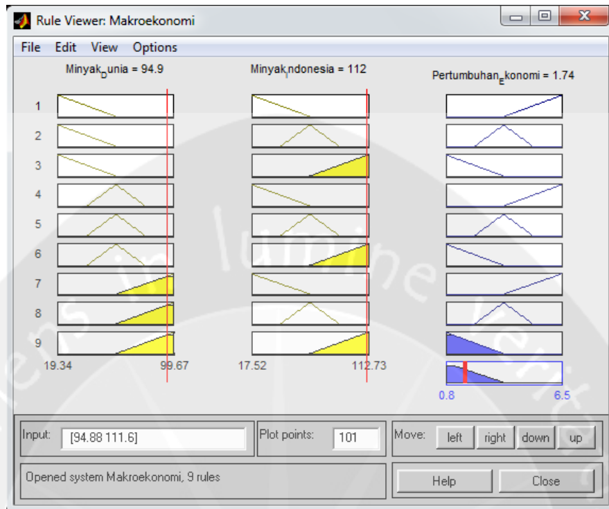
Lampiran 1.35 Deffuzifikasi tahun 2011
