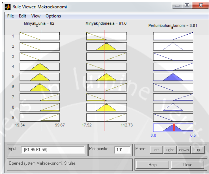
Lampiran 1.33 Deffuzifikasi tahun 2009
