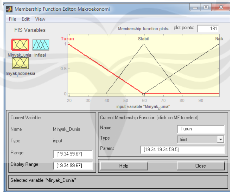
Lampiran 1.2 Himpunan Fuzzy Minyak Dunia
