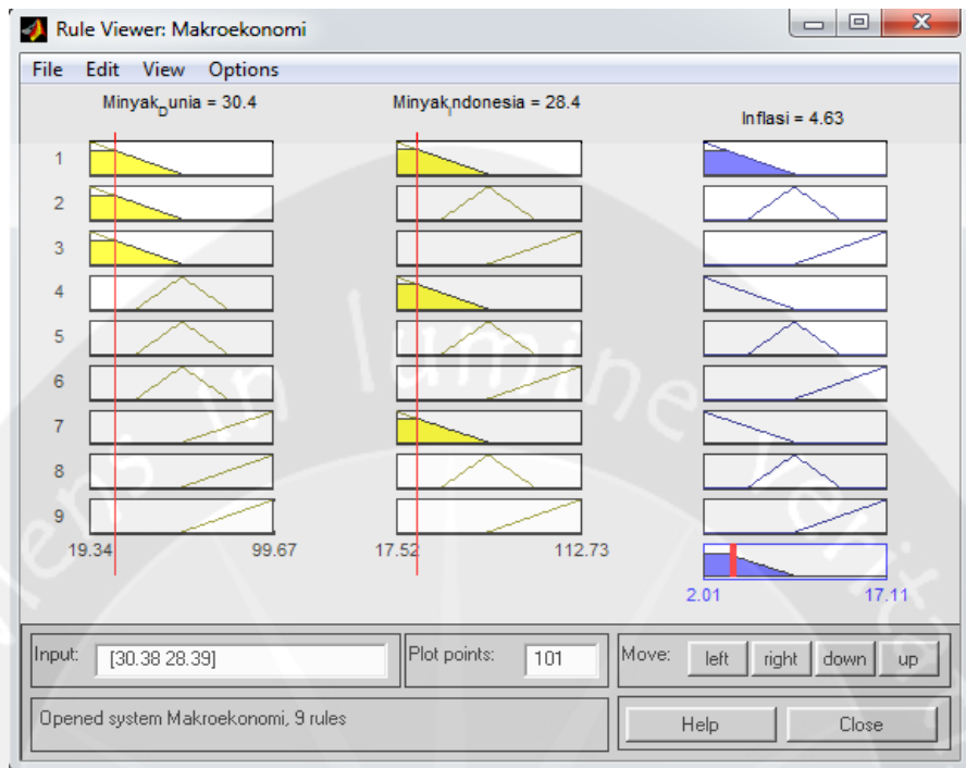
Lampiran 1.7 Deffuzifikasi tahun 2000
