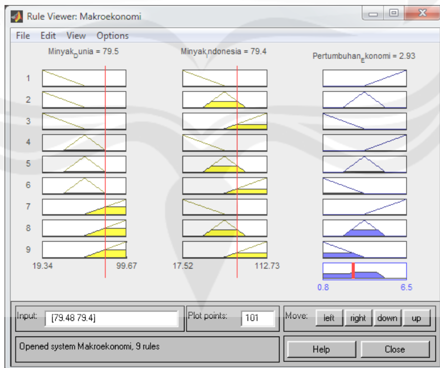
Lampiran 1.34 Deffuzifikasi tahun 2010
