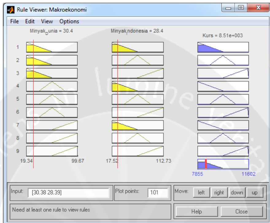
Lampiran 1.41 Deffuzifikasi tahun 2000
