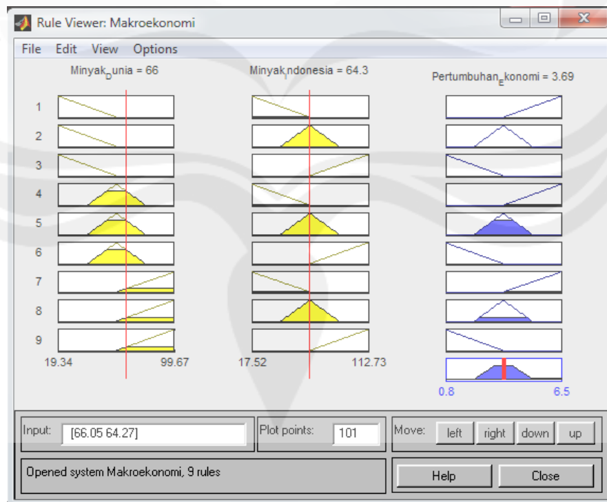
Lampiran 1.30 Deffuzifikasi tahun 2006
