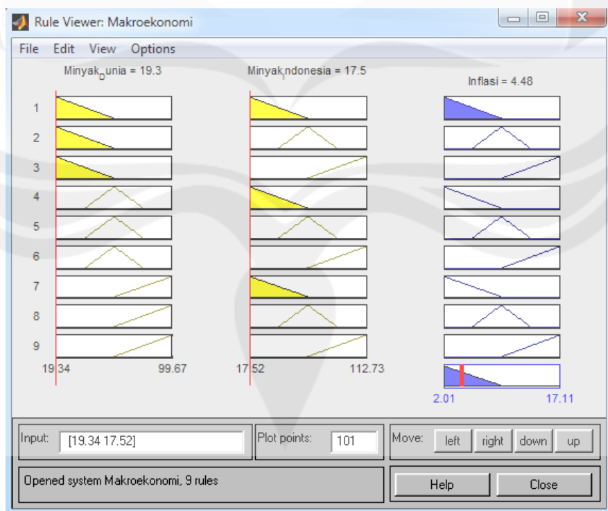
Lampiran 1.6 Deffuzifikasi tahun 1999
