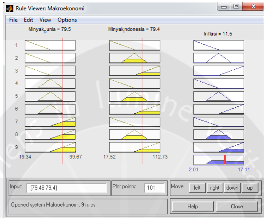
Lampiran 1.17 Deffuzifikasi tahun 2010
