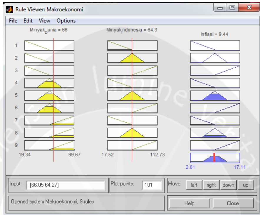
Lampiran 1.13 Deffuzifikasi tahun 2006
