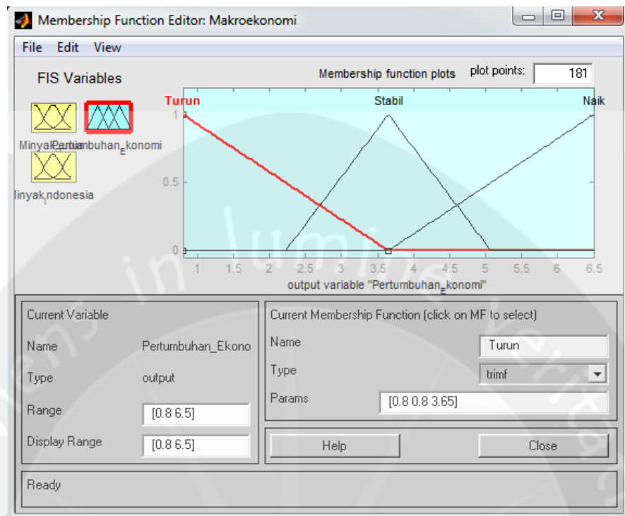
Lampiran 1.21 Himpunan Fuzzy Pertumbuhan ekonomi
