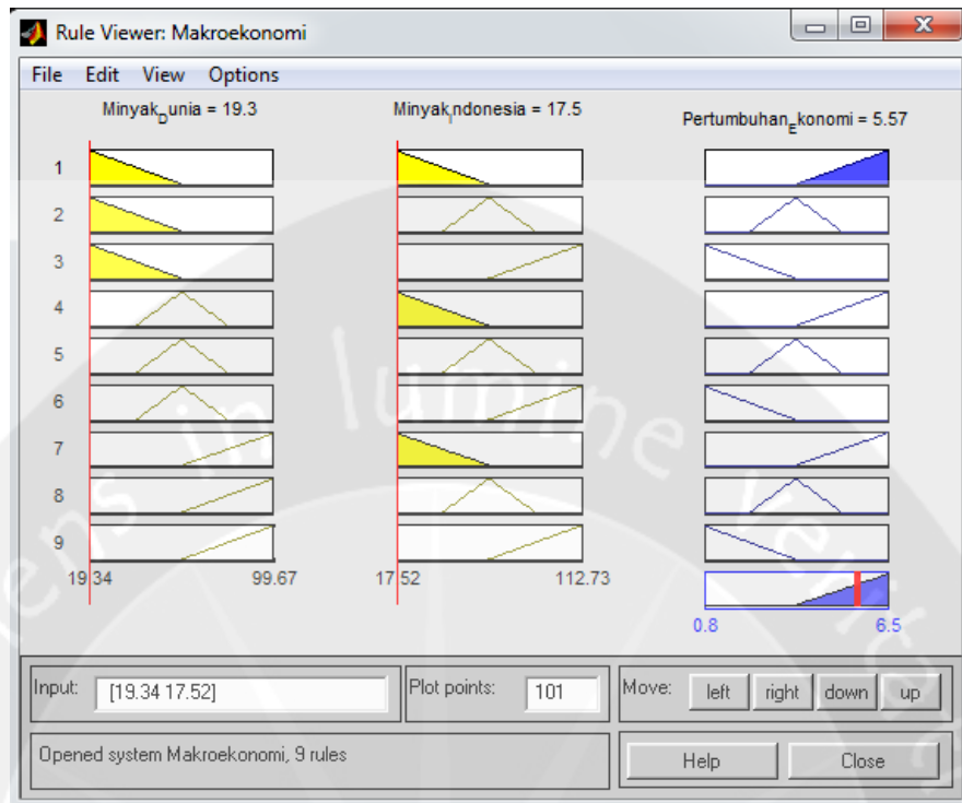
Lampiran 1.23 Deffuzifikasi tahun 1999
