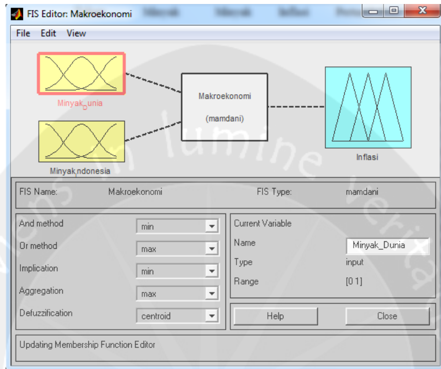
Lampiran 1.1 Variabel minyak dunia dan makroekonomi
