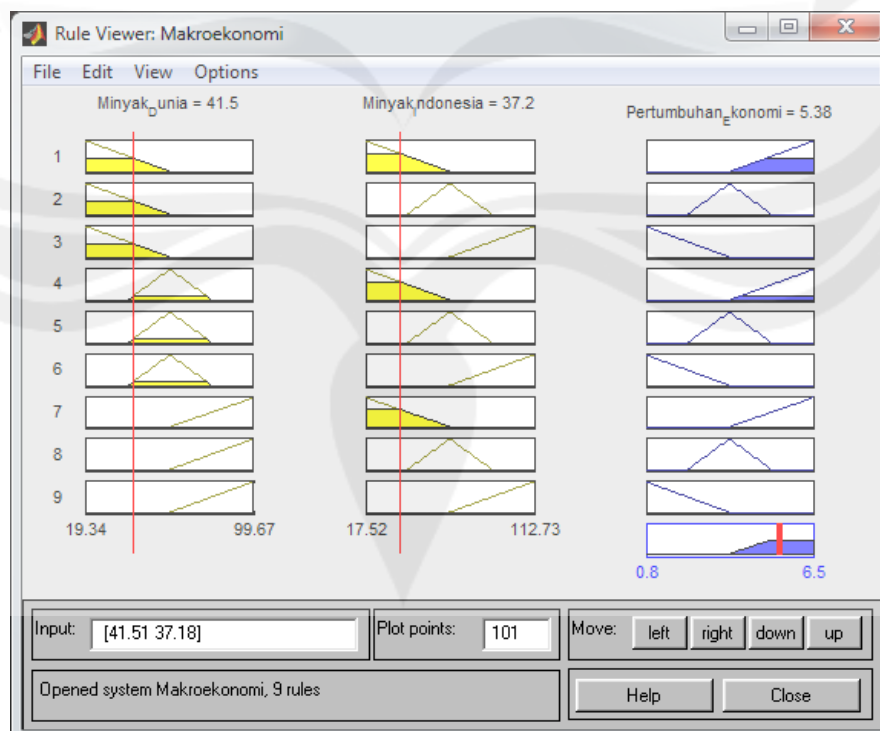
Lampiran 1.28 Deffuzifikasi tahun 2004
