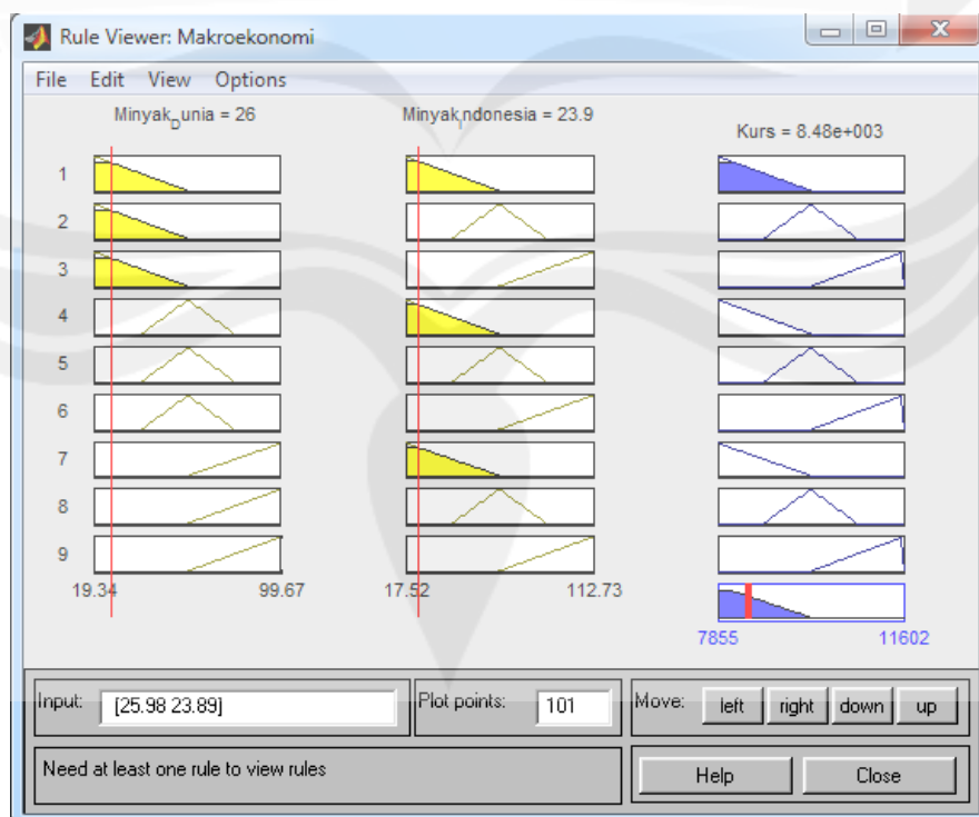
Lampiran 1.42 Deffuzifikasi tahun 2001
