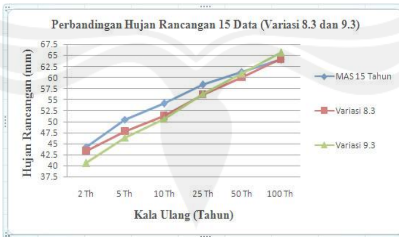
Gambar 9. Perbandingan Hujan Rancangan 15 data (Variasi 8.3 dan 9.3) dengan Tahun Awal 1986
