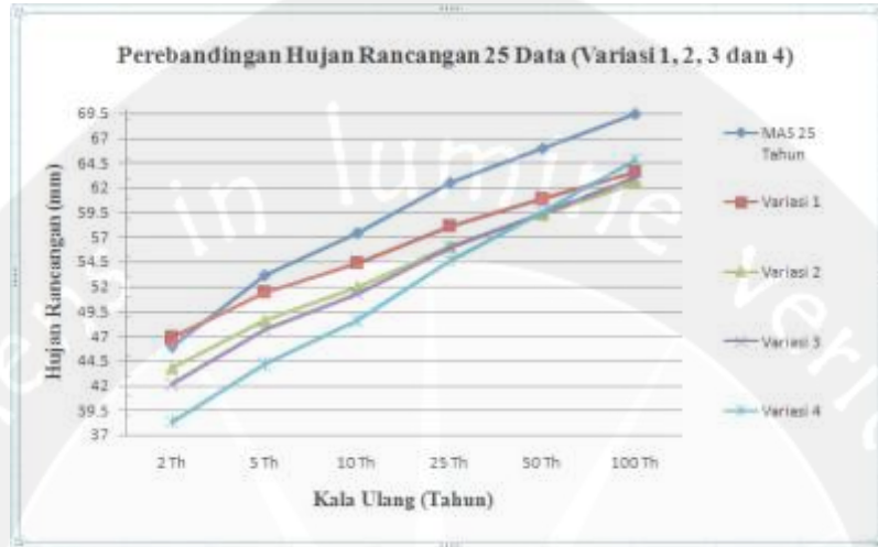
Gambar 1. Perbandingan Hujan Rancangan 25 Data (Variasi 1, 2, 3 dan 4)
