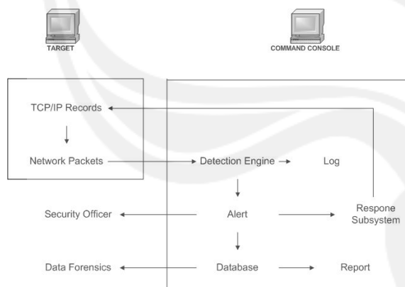
Gambar 2. Asitektur Standar NIDS (Anitha, 2011)
