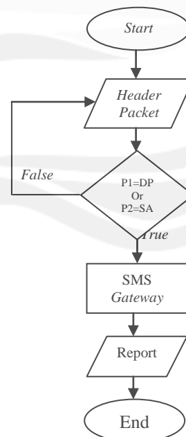
Gambar 4. Flowchart Penyaringan Data
