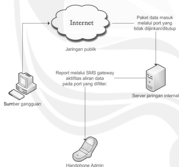
Gambar 6. Arsitektur Sistem
